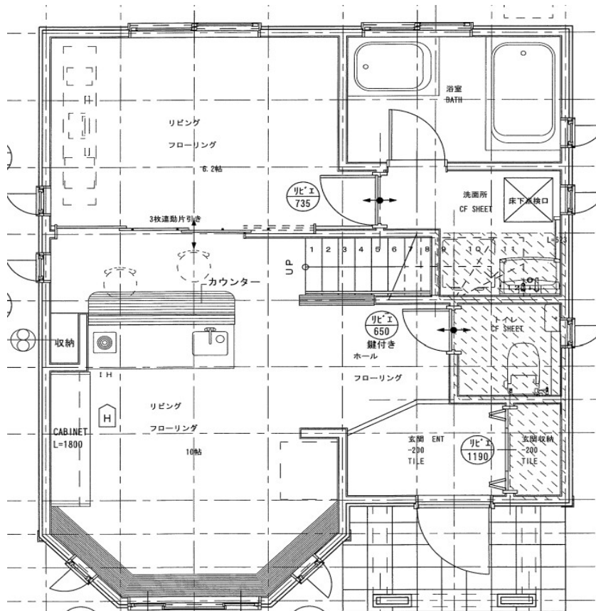
1階 平面図
