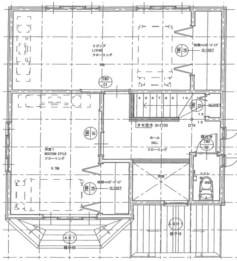
2階 平面図
