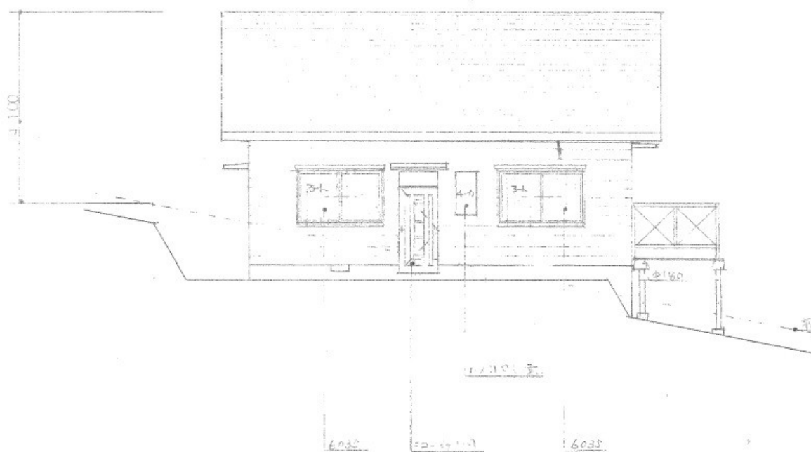
西立面図
