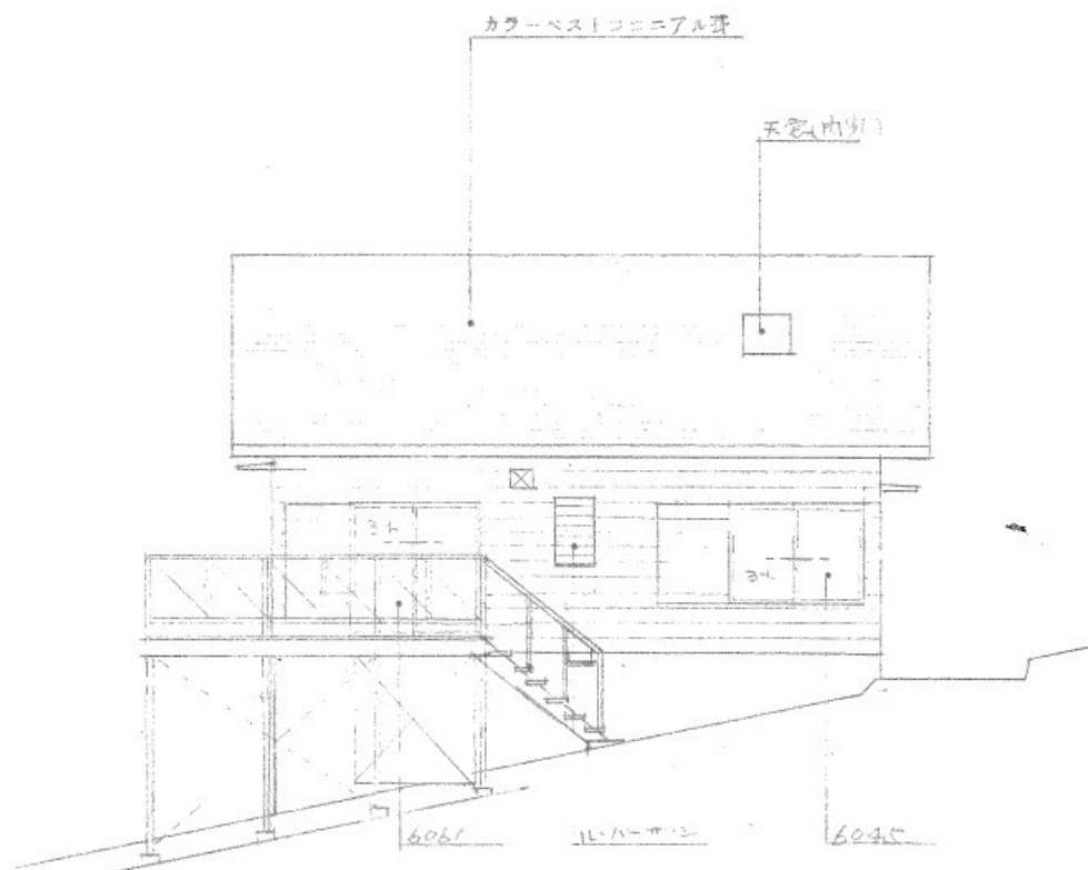
東立面図
