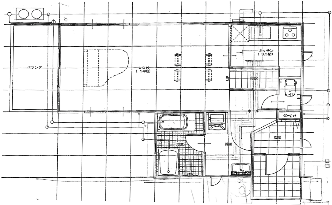
1階平面図
